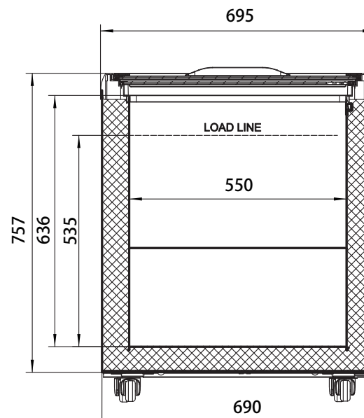
側面
