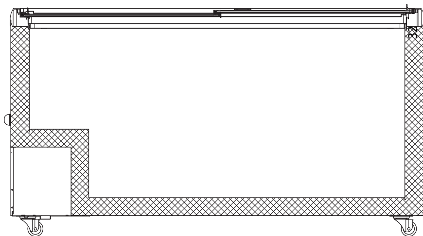
背面
