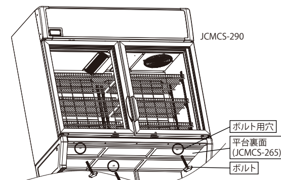
JCMCS-265 の平台に JCMCS-290 をボルトで固定する方法
